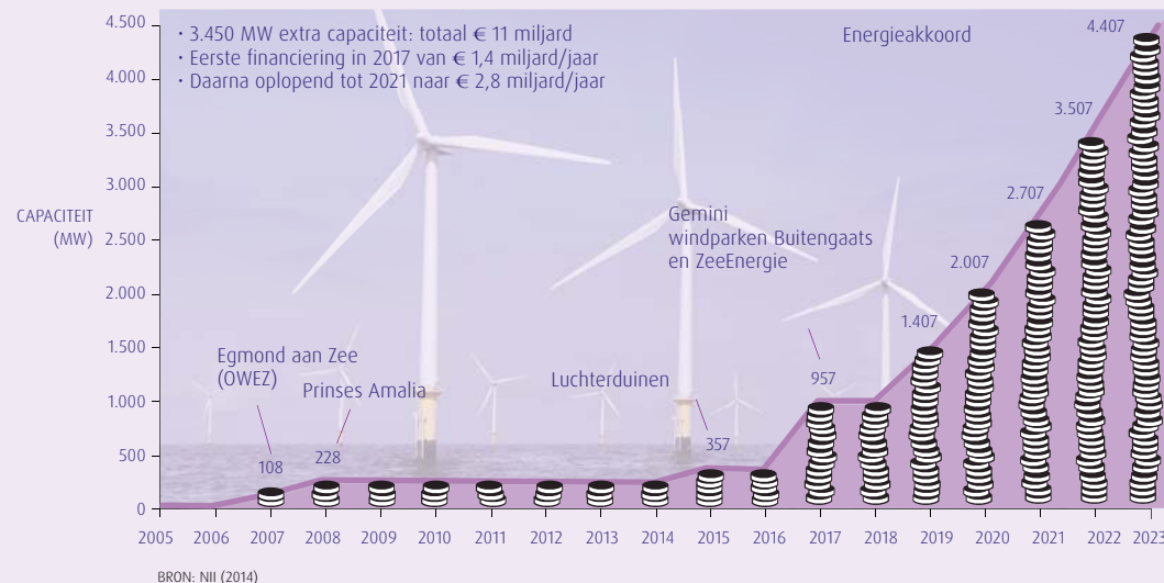
CUMULATIEF GEÏNSTALLEERD WIND-OP-ZEE-VERMOGEN EN KAPITAALBEHOEFTE IN NEDERLAND (MW, EURO)
