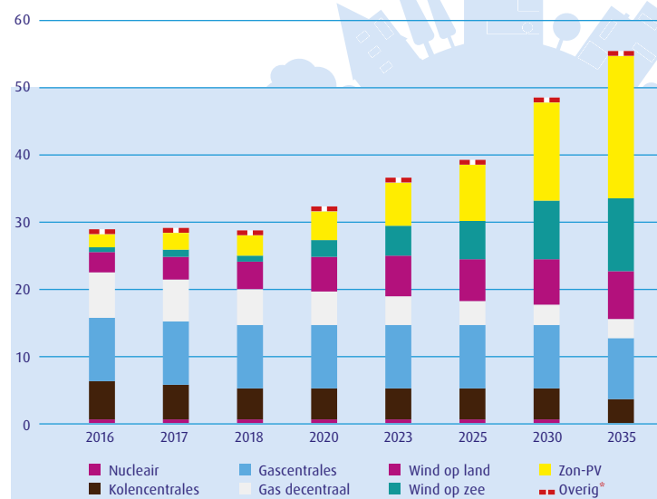
OPGESTELD VERMOGEN (gigawatt)
