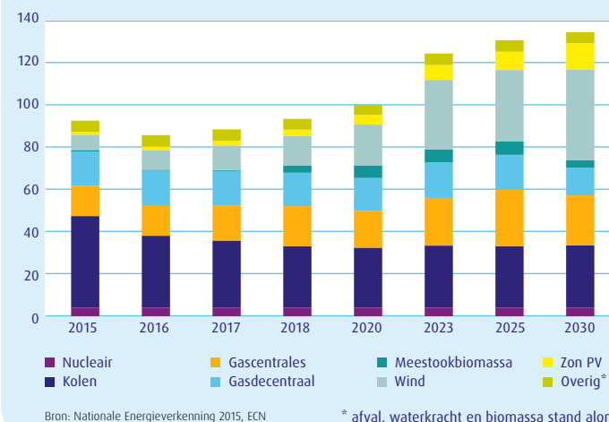
ONTWIKKELING VAN DE ELEKTRICITEITSPRODUCTIE NAAR ENERGIEDRAGER IN DE PERIODE 2015-2030
