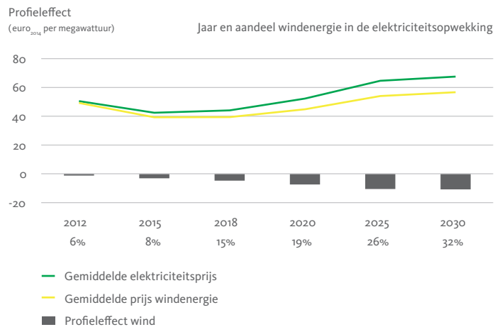
Figuur 4.6 Ontwikkeling van het profieffect op de prijs voor elektriciteit uit windenergie. Projectie bij vastgesteld beleid.
