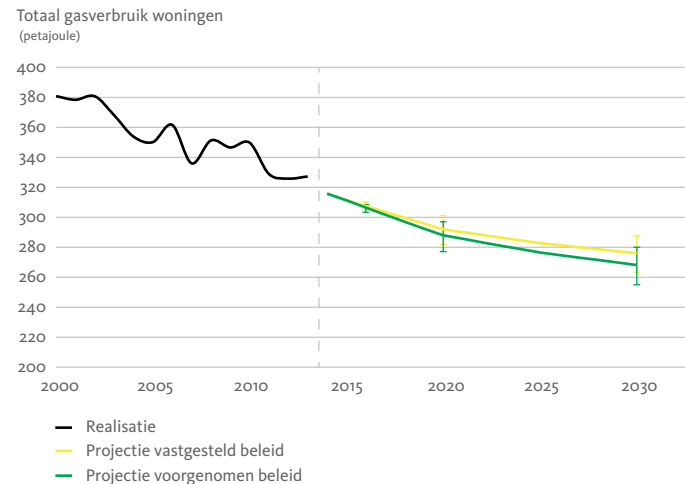
Figuur 5.2 Ontwikkeling van het aardgasverbruik door huishoudens, klimaatgecorrigeerd.
