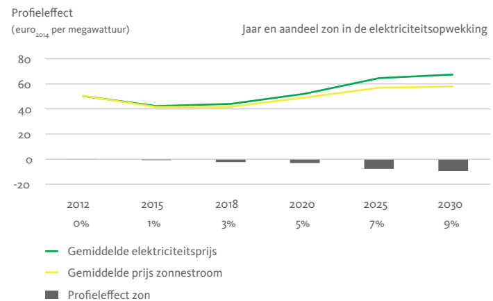
Figuur 4.7 Ontwikkeling van het profieffect op de prijs voor elektriciteit uit zonne-energie. Projectie bij vastgesteld beleid.
