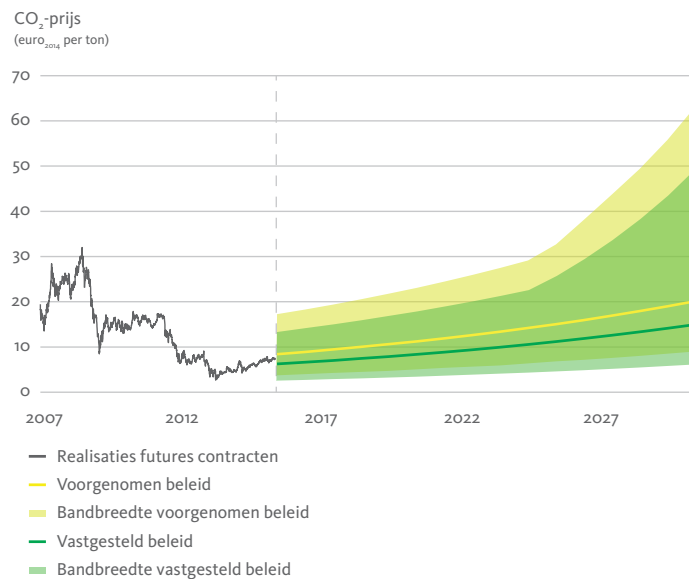
Figuur 2.9 Historische en geprojecteerde toekomstige prijzen voor CO 2 -emissierechten. Bron (voor realisatie): Point Carbon.
