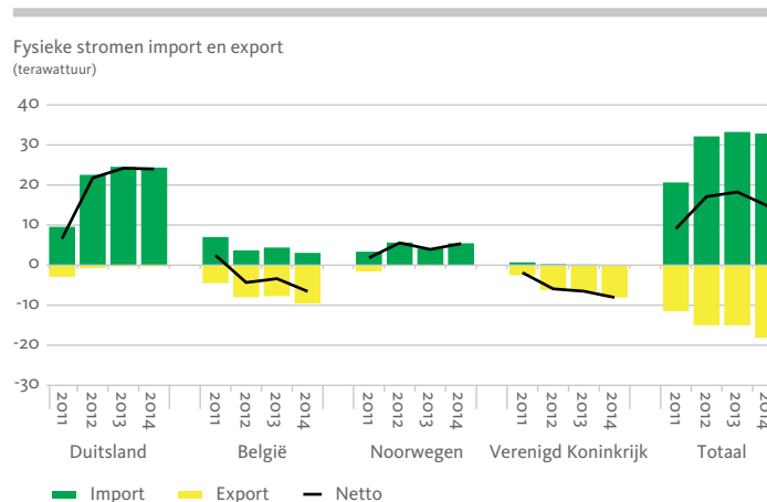
Figuur 2.7 Import en export van elektriciteit tussen Nederland en omliggende landen in de periode 2011-2014.
