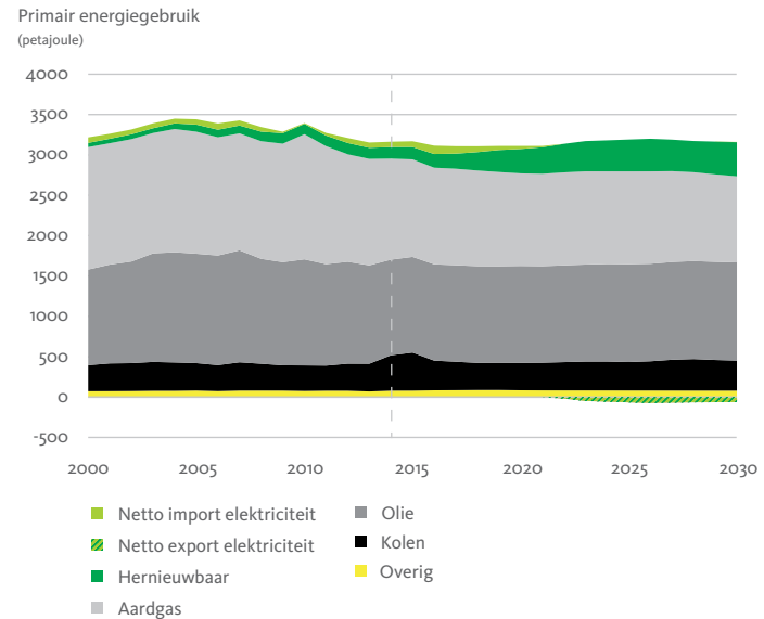
Figuur 3.6 Primair energiegebruik naar energiebron, temperatuurgecorrigeerd. Projectie bij voorgenomen beleid.
