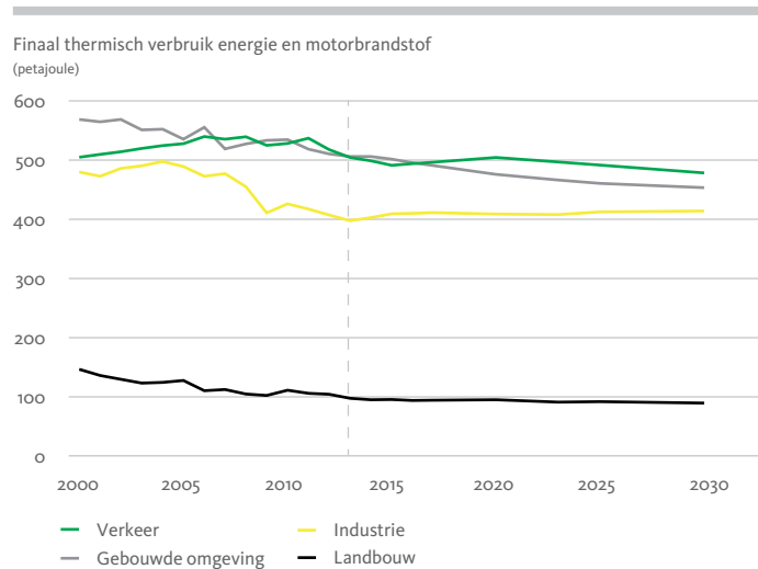
Figuur 3.3 Ontwikkeling van de vraag naar warmte en motorbrandstoffen door de verschillende eindverbruikers in de periode 2000-2030. Projectie bij voorgenomen beleid.
