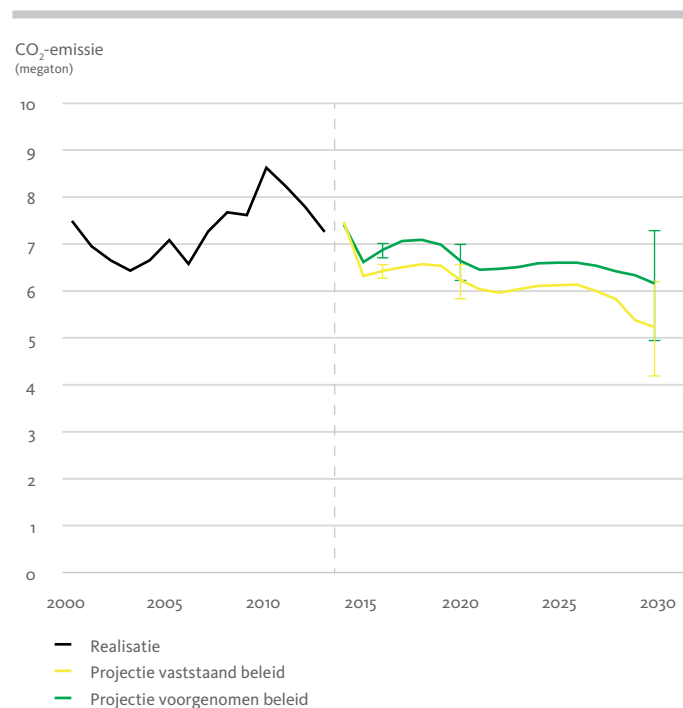
Figuur 5.17 Ontwikkeling van de CO 2 -emissies in de landbouw in de periode 2000-2030.
