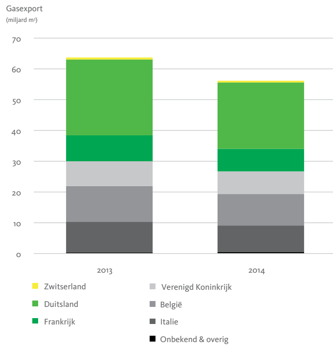
Figuur 4.11-b Bestemming van gasexport in 2013 en 2014.
